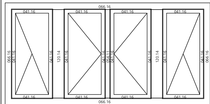
Typ 18) Fenster vierflügelig mit 2 Setzhölzern und einer Schlagleiste
