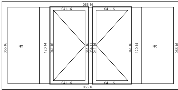
Typ 19) Fenster vierteilig mit 2 Setzhölzern und einer Schlagleiste, links und rechts FIX
