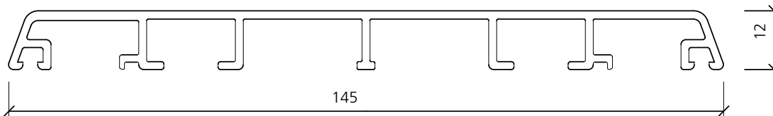
145.12 Setzprofil
