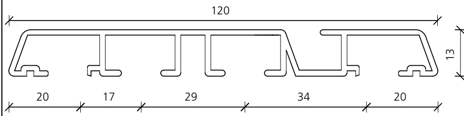
120.13 Kämpferprofil
