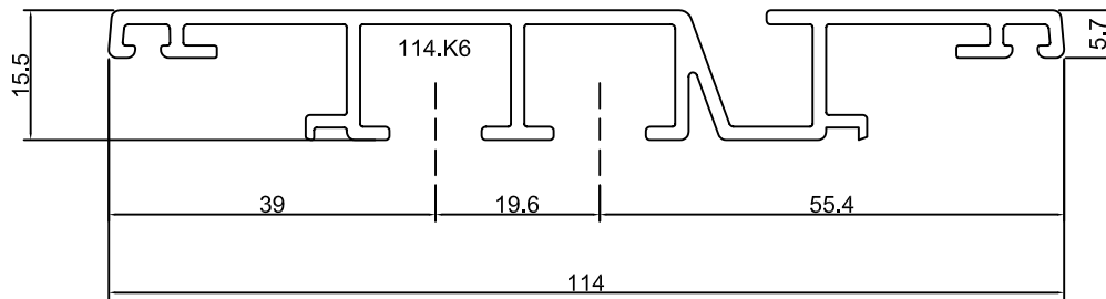
114.K6 Kämpfer
