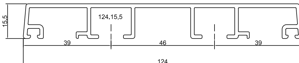
124.15,5 Setzholz
